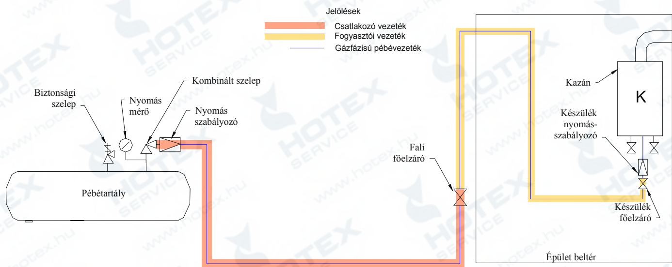
7.1.2.2. sz. ábra A csatlakozó és a fogyasztói vezeték egyszerű pébégáz ellátó rendszerénél
