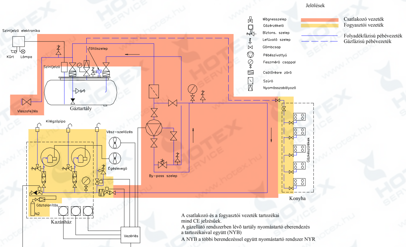
7.1.2.4. sz. ábra A csatlakozó és a fogyasztói vezeték határai szivattyús és egyszerű pégáz ellátó rendszernél
