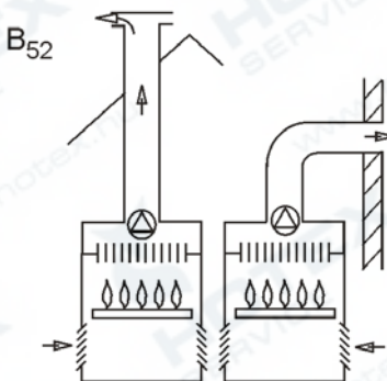
Ventilátor a tüztér/ hőcserélő után
