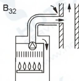
Ventilátor a tüztér/ hőcserélő után
