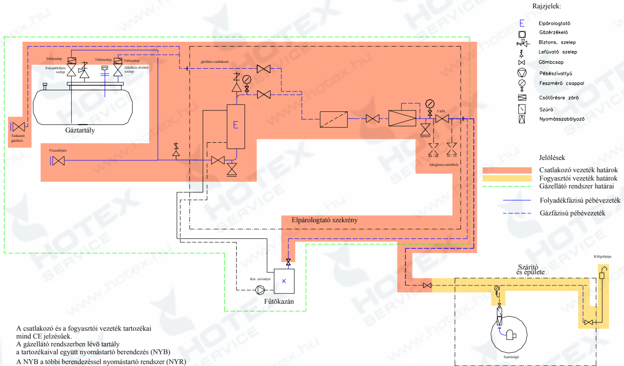
7.1.2.3. sz. ábra A csatlakozó és a fogyasztói vezeték határai elpárolgató pégáz ellátó rendszernél
