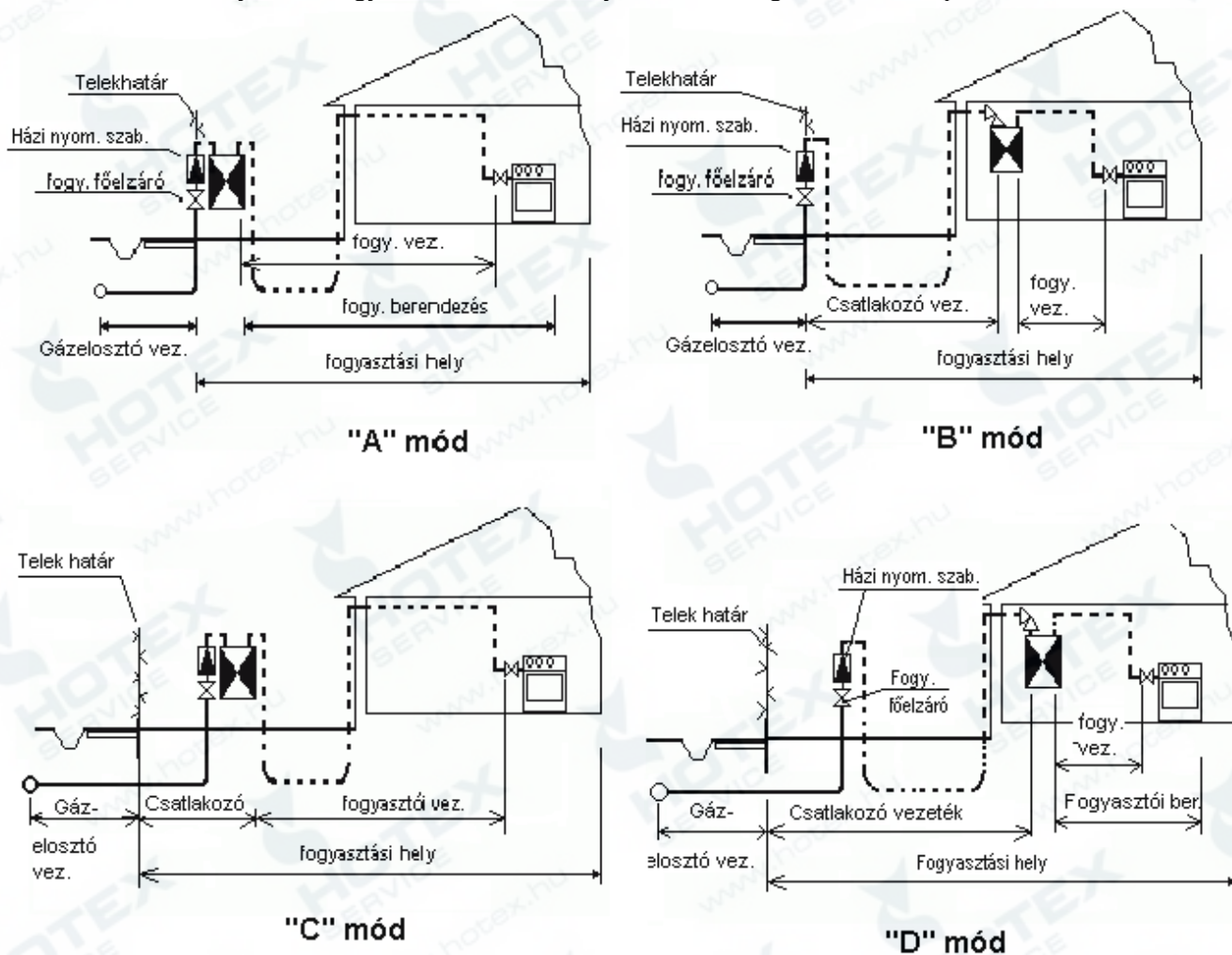
7.1.1.2. sz. ábra A kisnyomású fogyasztói főelzáró elhelyezési lehetőségei zárt sorú beépítés esetén
